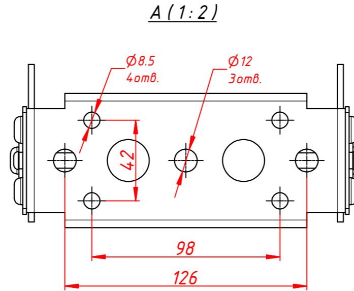
Точки крепления
