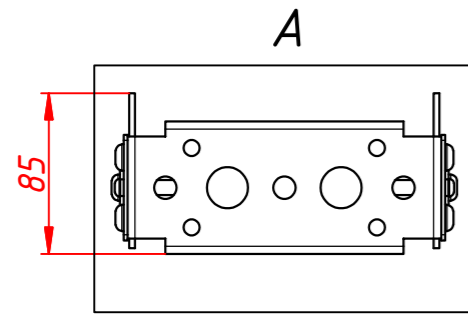
Габаритные размеры
